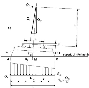
Fig. 5.2.6 - Distribuzione trasversale in curva delle azioni per mezzo delle traverse e del ballast. In figura, Q_f rappresenta la forza centrifuga definita al successivo §5.2.2.3.1
